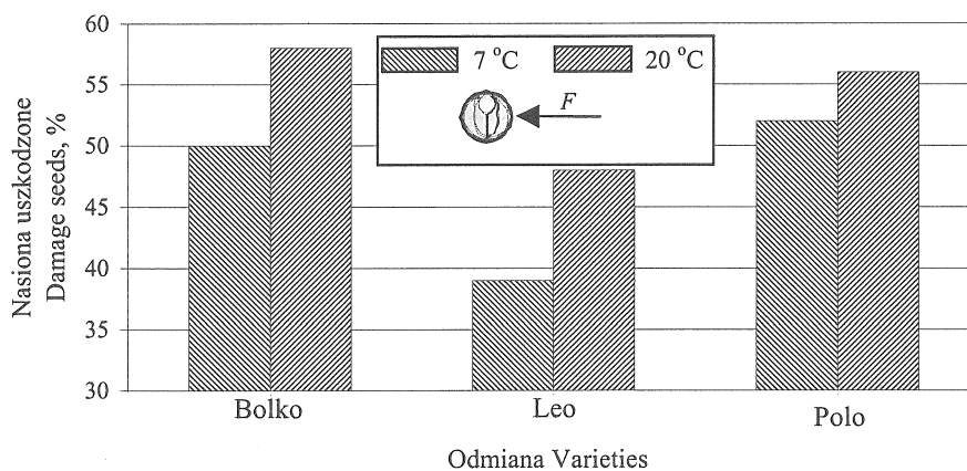
Rys. 2. Zależność, procent uszkodzeń – odmiana, dla nasion rzepaku przechowywanych w warunkach laboratoryjnych przez 180 dni w temperaturze powietrza 7 i 20°C
